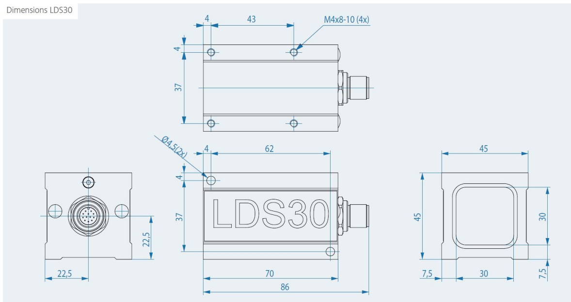
Dimensions LDS30
